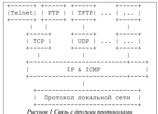
Рисунок 1 Связь с другими протоколами
