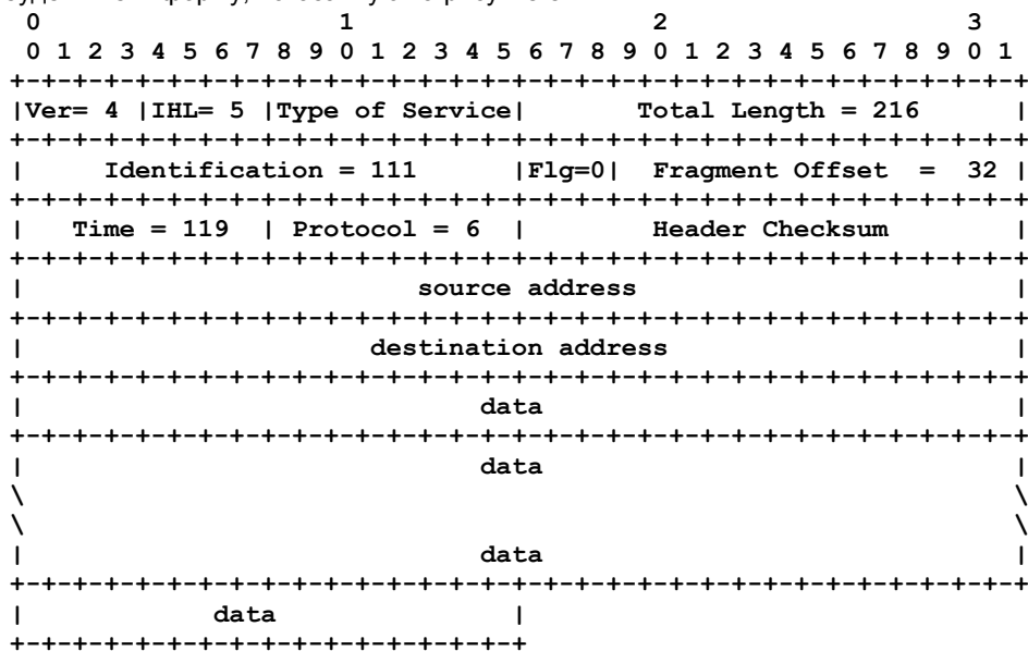
Рисунок 8. Пример фрагмента дейтаграммы IP.
