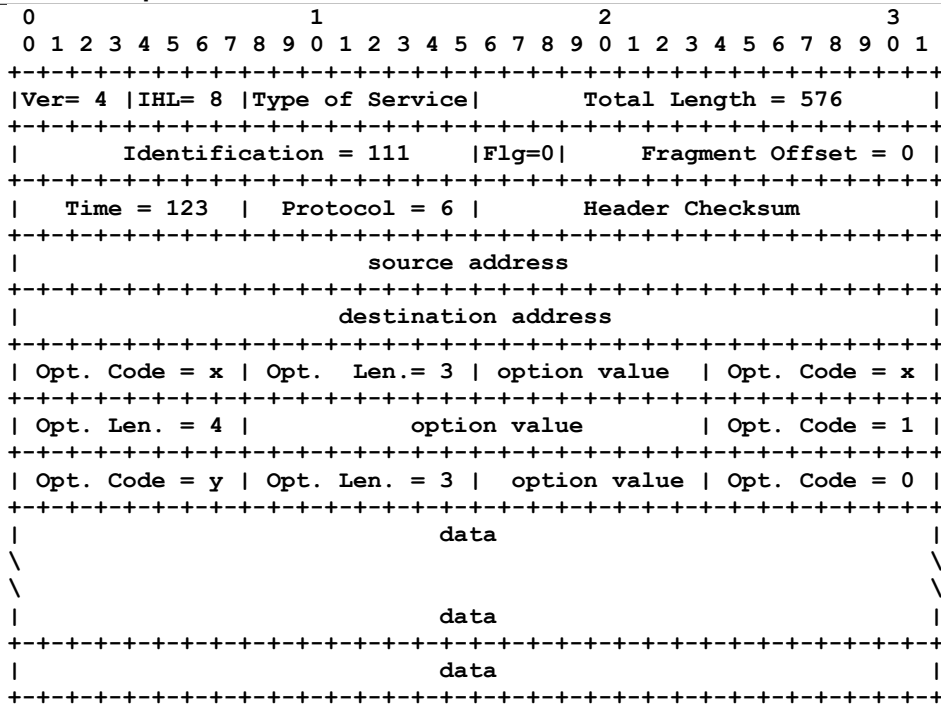
Рисунок 9. Пример дейтаграммы IP с опциями.
