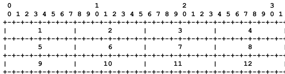
Рисунок 10. Порядок передачи байтов.
