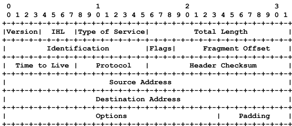
Рисунок 4. Формат заголовка дейтаграммы IP.
