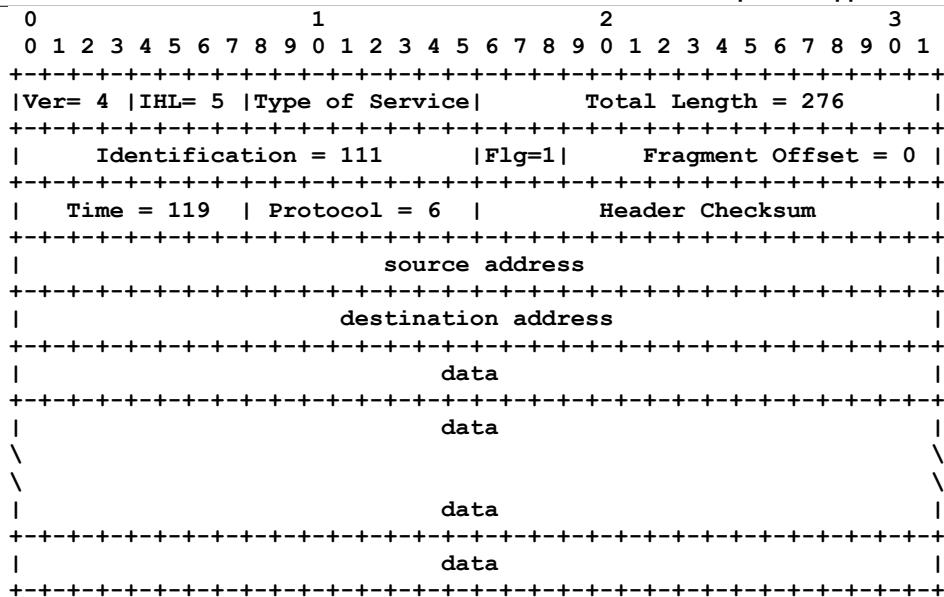
Рисунок 7. Пример первого фрагмента дейтаграммы IP.
