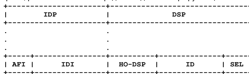
Рисунок 1. Иерархическая структура адресов ISO.
