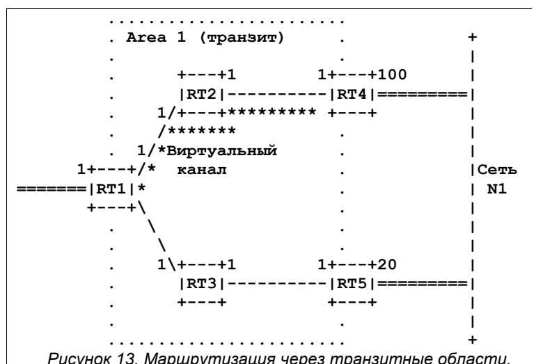
Рисунок 13. Маршрутизация через транзитные области.
