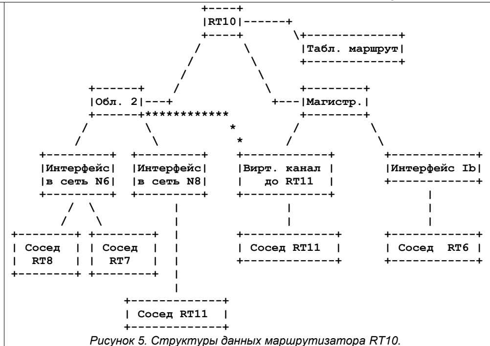
Рисунок 5. Структуры данных маршрутизатора RT10.
