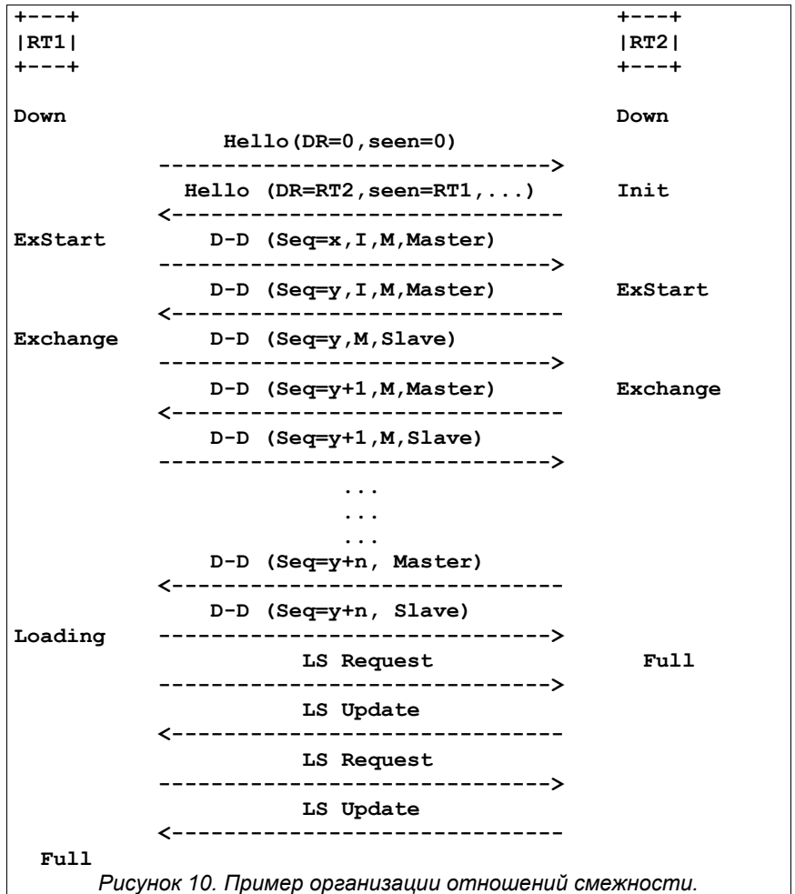
Рисунок 10. Пример организации отношений смежности.
