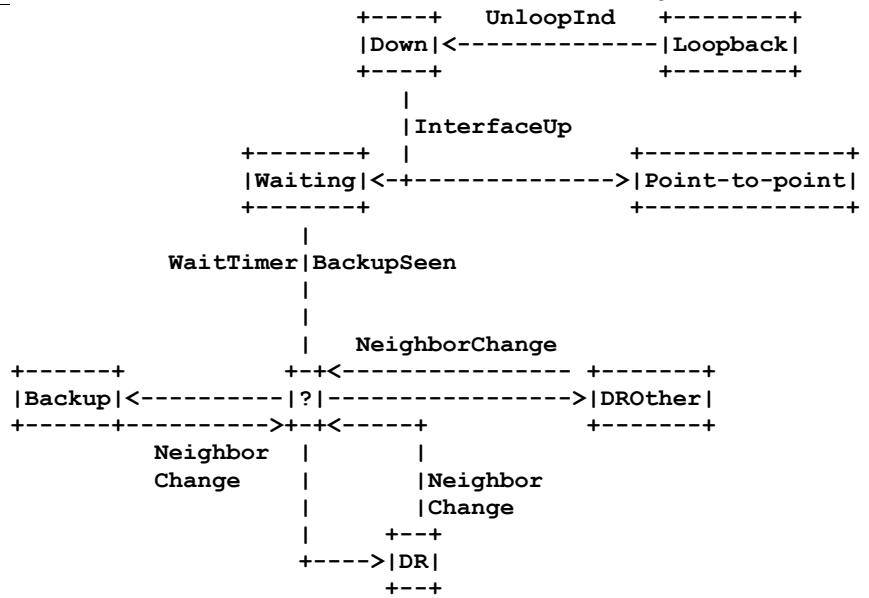
Рисунок 7. Смена состояния интерфейса В дополнение к показанным на графе переходам событие InterfaceDown всегда приводит к состоянию Down, а LoopInd – к состоянию Loopback.
