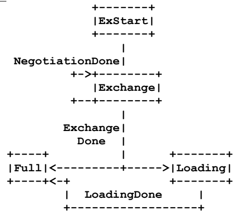
Рисунок 9. Смена состояний соседа (Database Exchange)
