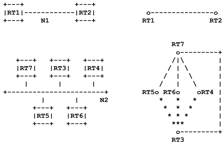
Рисунок 6. Граф смежности
