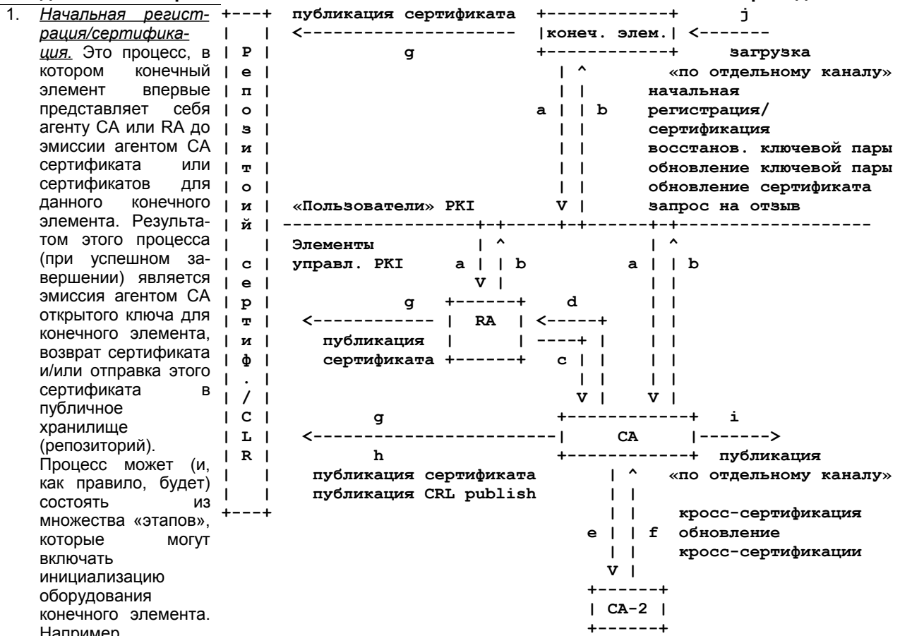
Рисунок 1: Элементы PKI
