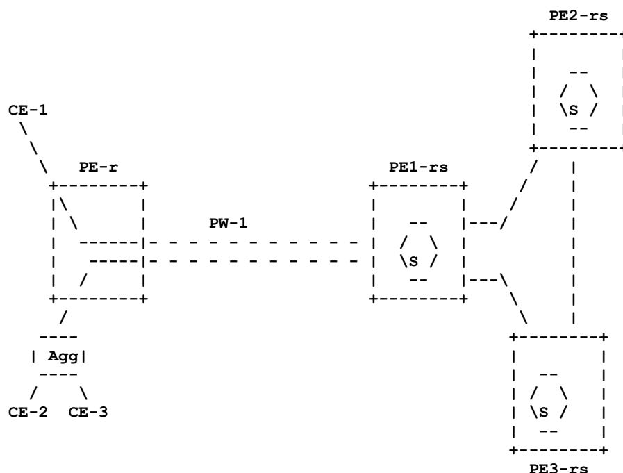
Рисунок 4. Пример иерархической VPLS с лучами без мостов.
