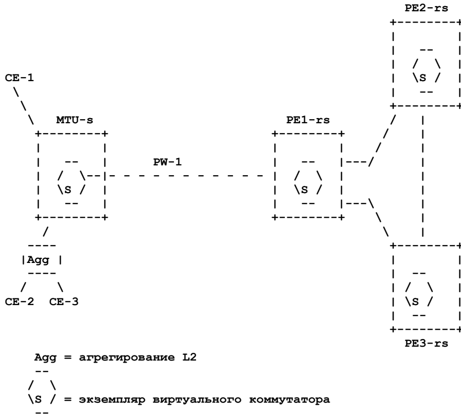
Рисунок 3. Пример иерархической модели VPLS.
