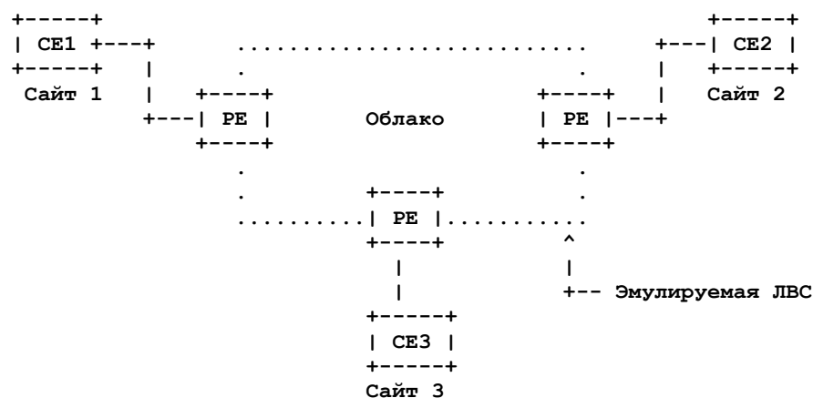
Рисунок 1. Топологическая модель VPLS для абонента с 3 сайтами.
