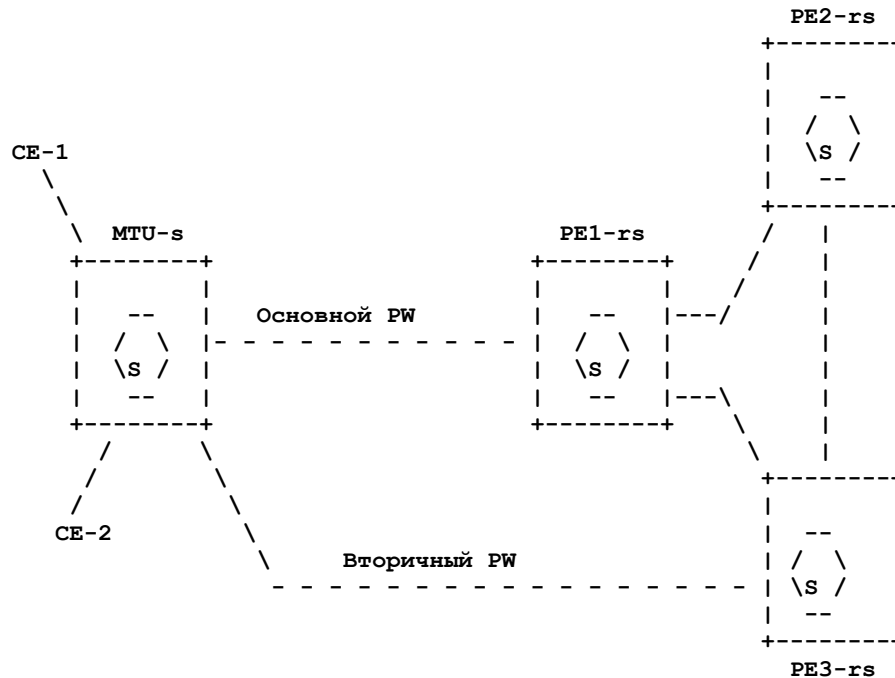
Рисунок 5. Пример двудомного MTU-s.
