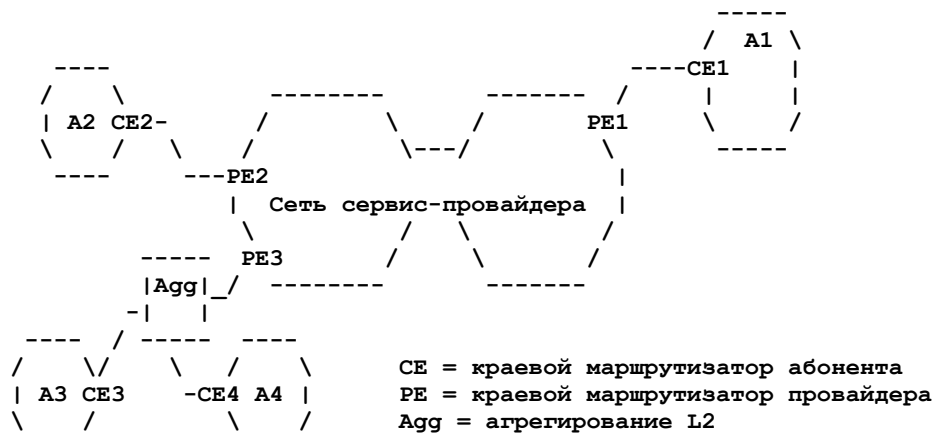
Рисунок 2. Пример VPLS.
