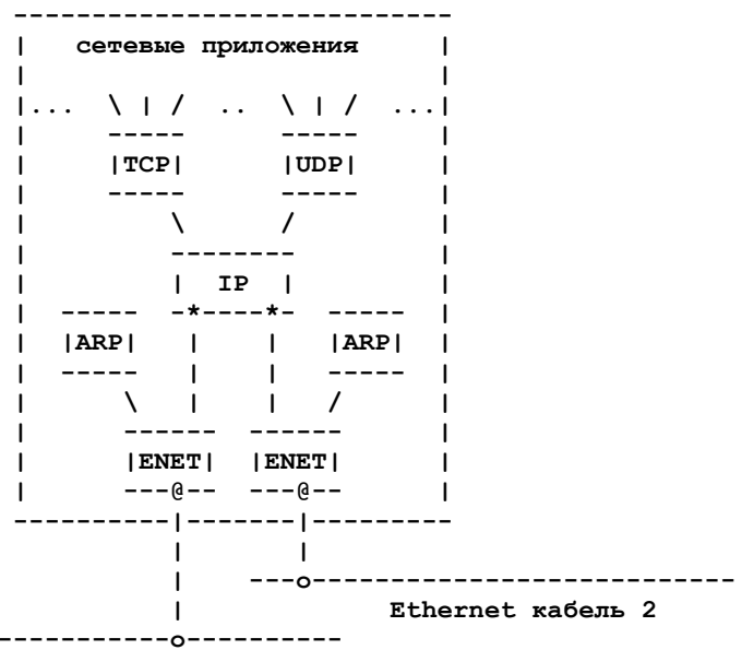
Рисунок 3. Узел сети TCP/IP с двумя адаптерами Ethernet
