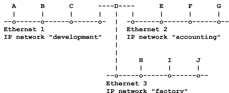
Рисунок 7. Три сети IP в одной сети internet
