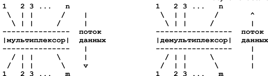
Рисунок 4. Мультиплексор и демультиплексор n x m
