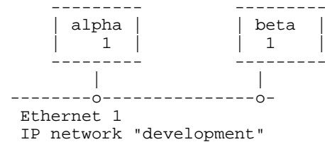
Рисунок 8. Фрагмент IP-сети
