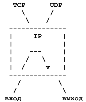
Рисунок 5. Пример пересылки пакета IP (IP Forwarding)
