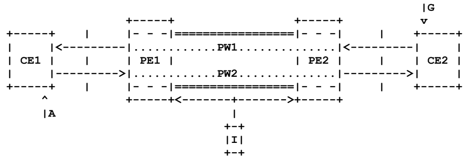
Рисунок 4: Сценарий с синхронизацией через сеть PSN
