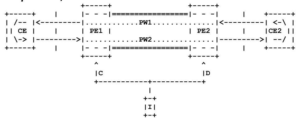
Рисунок 2: Сценарий синхронизации PE
