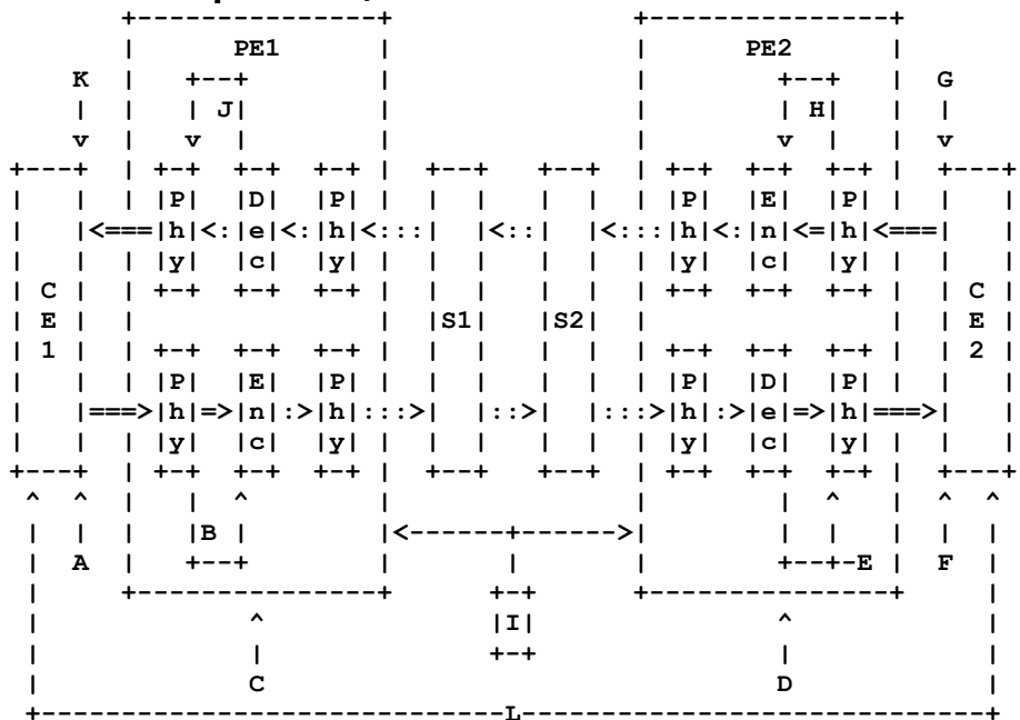
Рисунок 1: Эталонная модель сетевой синхронизации
