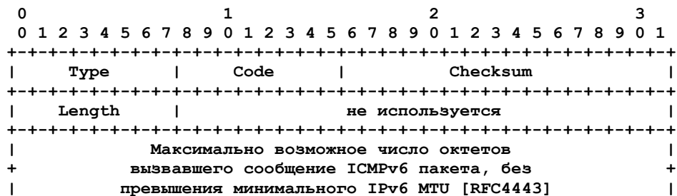
Рисунок 4. ICMPv6 Destination Unreachable
