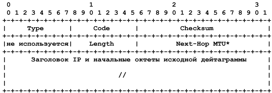
Рисунок 1. ICMPv4 Destination Unreachable
