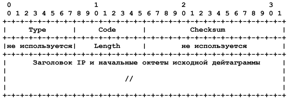
Рисунок 2. ICMPv4 Time Exceeded
