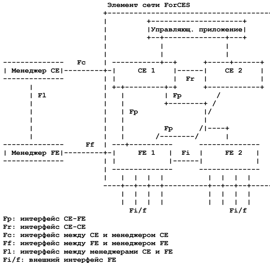
Рисунок 1. Архитектурная схема ForCES.
