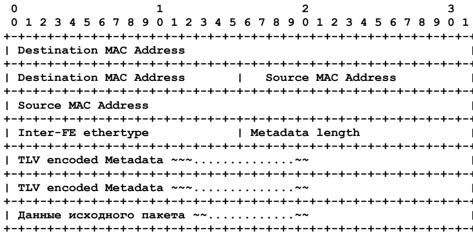
Рисунок 6. Формат пакета.
