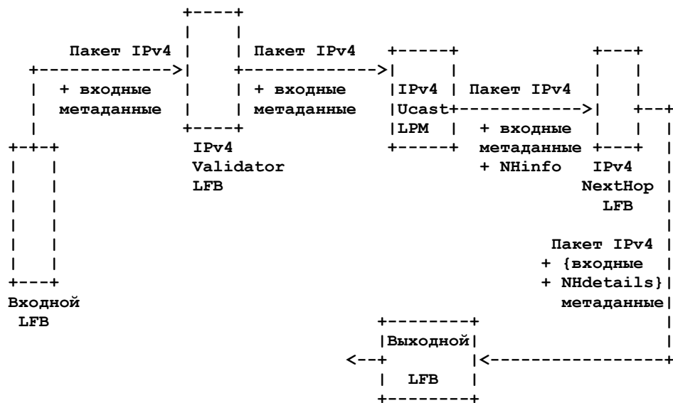
Рисунок 1: Топология LFB базового обслуживания пакетов IPv4.
