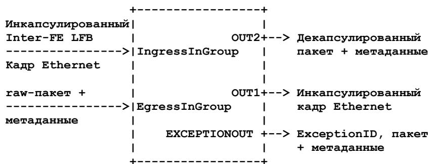
Рисунок 7. Inter-FE LFB.
