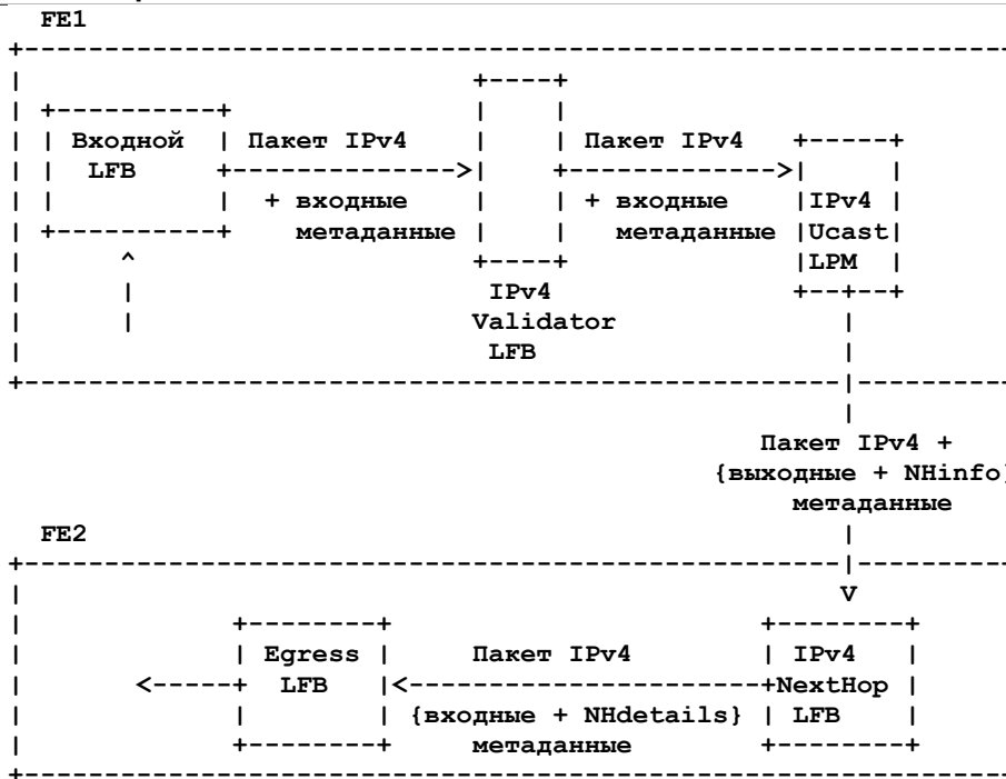
Рисунок 2. Расщепление топологии LFB для обслуживания пакетов IPv4.
