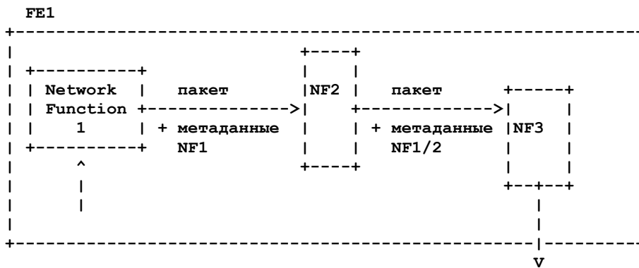
Рисунок 3. Цепочка сетевых функций внутри одного FE.
