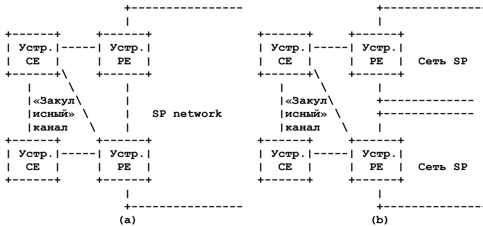
Рисунок 4. Комбинация двудомных подключений и "закулисных" канала для CE.
