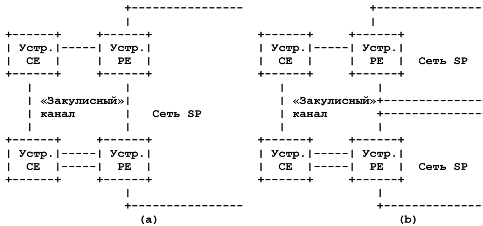
Рисунок 3. «Закулисные» соединения между CE.
