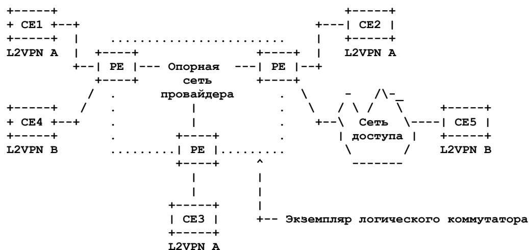
Рисунок 1. Эталонная модель L2VPN.
