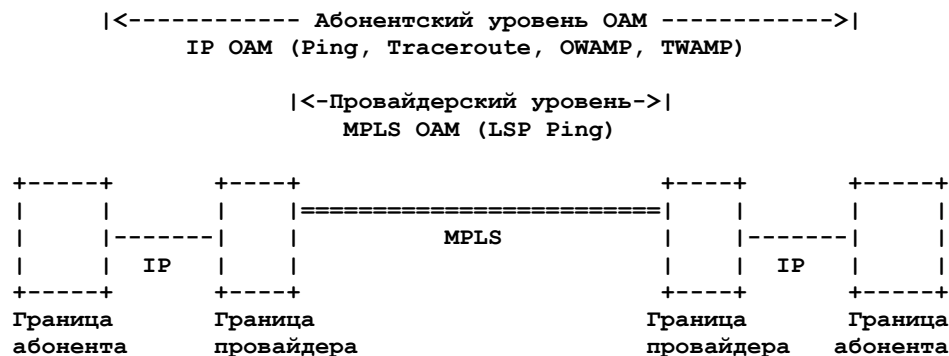
Рисунок 1. Пример многоуровневой организации OAM.
