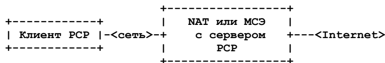
Рисунок 1. Межсетевой экран или устройство NAT с поддержкой PCP.
