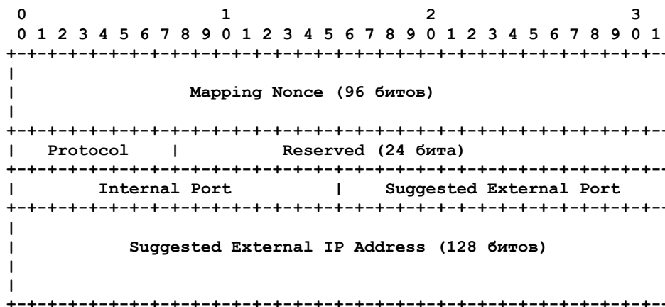
Рисунок 9. Запрос MAP.
