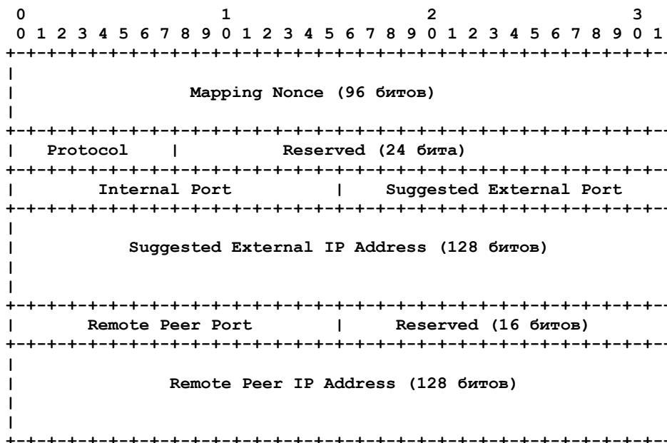
Рисунок 11. Запрос PEER.
