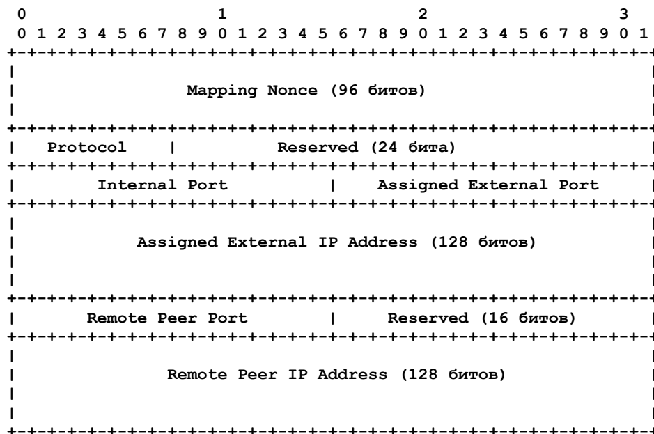
Рисунок 12. Отклик PEER.
