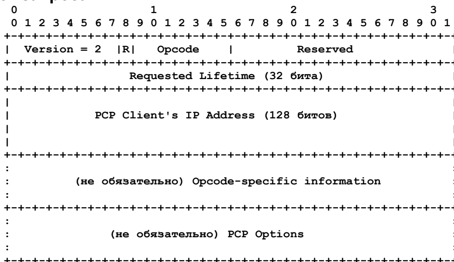
Рисунок 2. Формат запроса.
