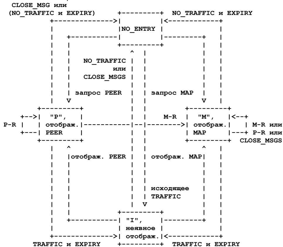
Рисунок 16. Диаграмма состояний PCP.
