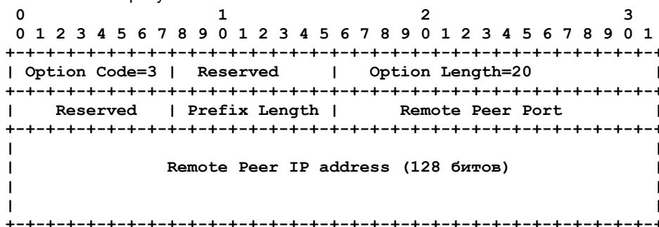
Рисунок 15. Схема опции FILTER.
