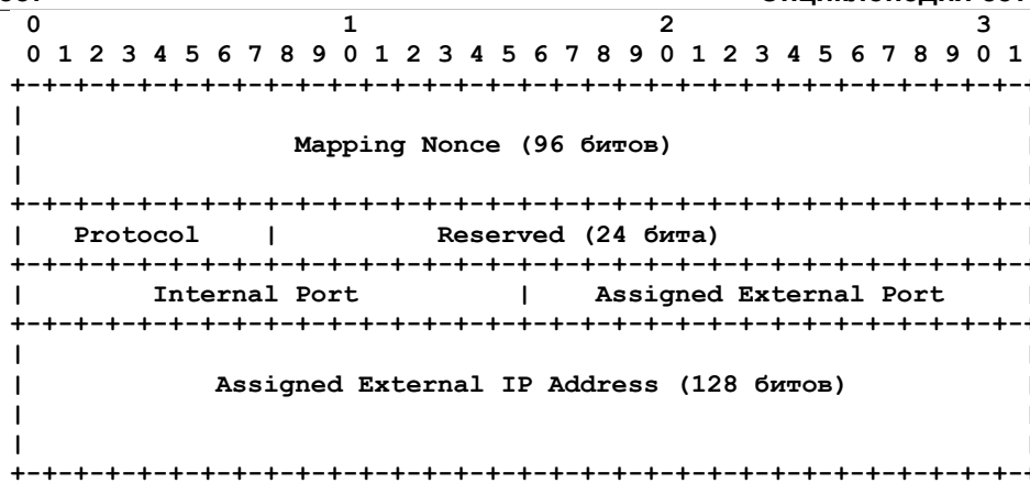
Рисунок 10. Отклик MAP.
