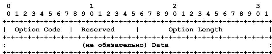
Рисунок 4. Заголовок опций.
