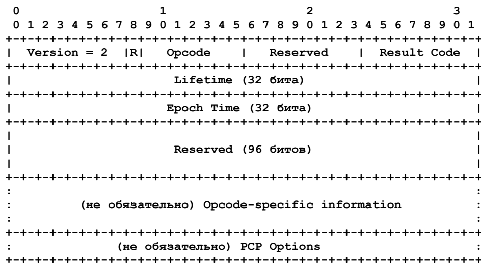
Рисунок 3. Формат отклика.
