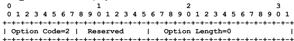
Рисунок 14. Опция PREFER_FAILURE.
